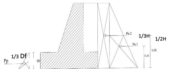
Gambar 5. Tekanan Lateral Tanah Sumber : Hardiyatmo, 2020
