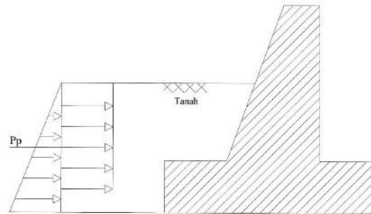
Gambar 11. Tekanan Tanah Pasif Sumber: Hardiyatmo, 2020
