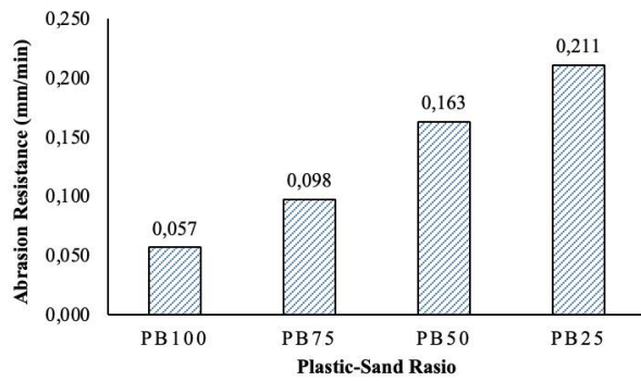
Gambar 12. Rata-rata ketahanan aus paving block dengan variasi rasio plastik-pasir
