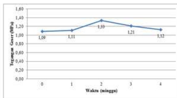
Gambar 6. Grafik pengaruh perendaman air laut terhadap tegangan geser interfacial
