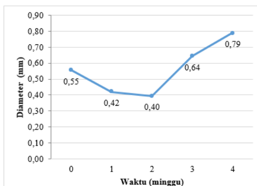
Gambar 4. Grafik pengaruh perendaman air laut terhadap diameter serat
