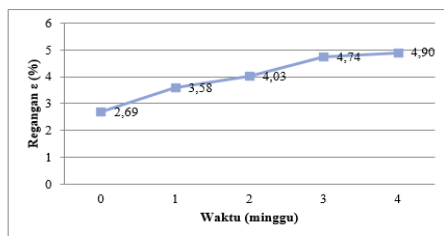
Gambar 3. Grafik pengaruh perendaman air laut terhadap regangan serat
