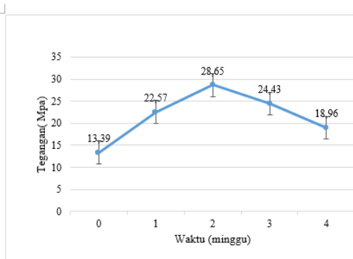
Gambar 2. Grafik pengaruh perendaman air laut terhadap tegangan tarik
