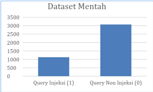
■ Gambar 4 Dataset sebelum diterapkan SMOTE.
