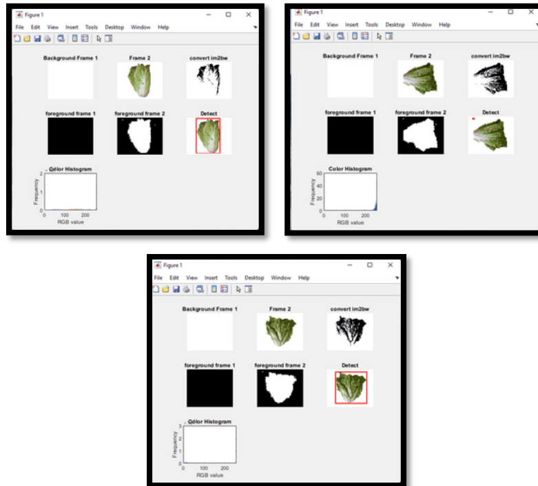
Gambar 2. Deteksi Objek
