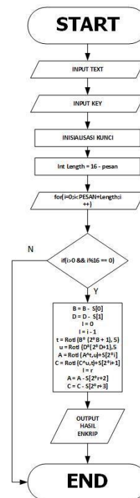
Gbr 10 Diagram Alur Algoritma Enkripsi RC6
