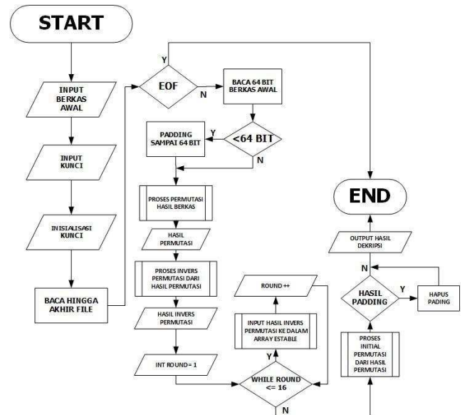
Gbr 15 Diagram Alur Algoritma Dekripsi DES
