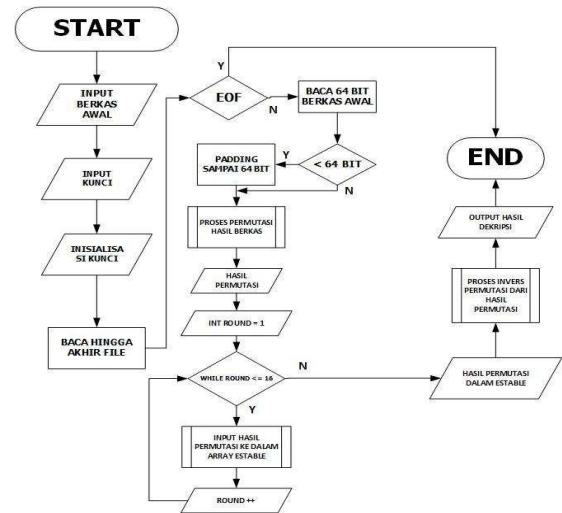
Gbr 14 Diagram Alur Algoritma Enkripsi DES
