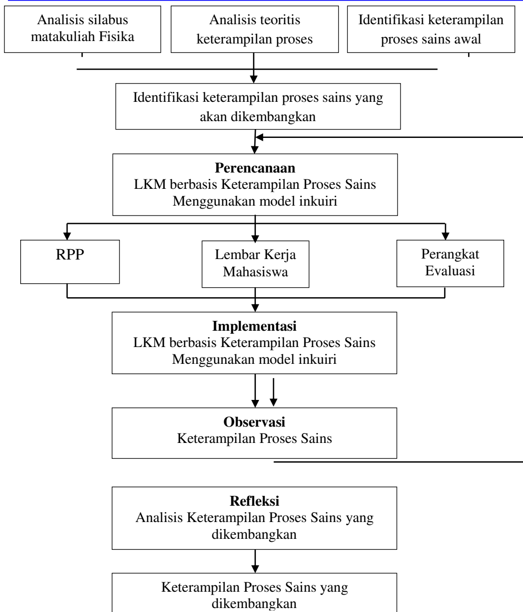
Gambar 1. Desain Penelitian
