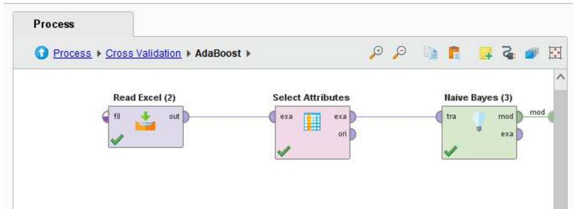
Gambar 6. Implementasi Naïve Bayes dengan Adaboost
