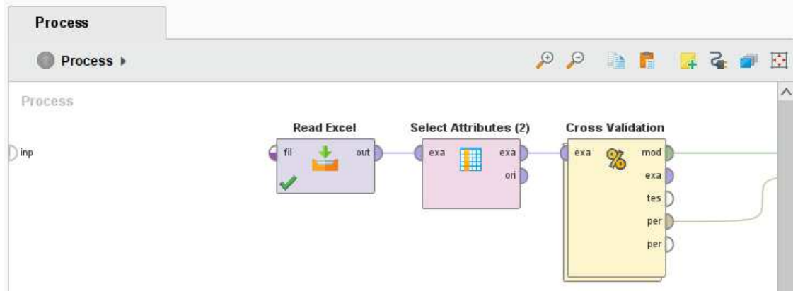
Gambar 3. Tahap Validasi
