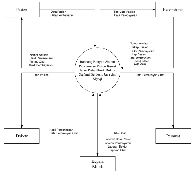
Gambar 1 Diagram Konteks
