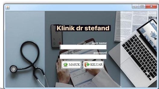
Gambar 9 Login
