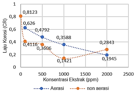
Gambar 3. Hubungan antara konsentrasi ekstrak dan kondisi lingkungan dengan laju korosi
