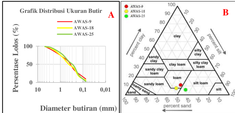
Gambar 3. Karakteristik tanah: (A) Prosentase vs diameter ukuran butir, dan (B) Jenis tanah berdasarkan distribusi ukuran butir pada klasifikasi USDA
