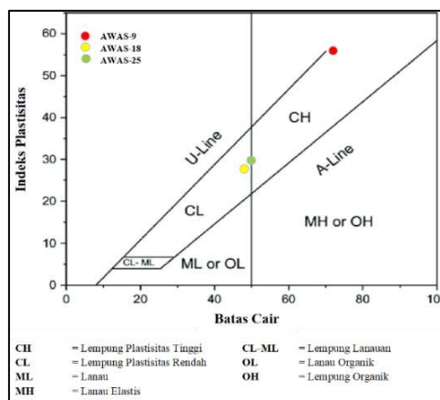
Gambar 4. Hasil uji Atterberg limit pada grafik plastisitas
