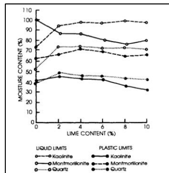
Gambar 9. Batas cair dan batas plastis dari kaolinit, montmorillonit, dan kuarsa pada prosentase penambahan batukapur dan moisture content yang bervariasi [20]
