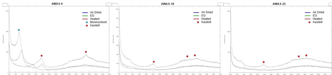
Gambar 5. Grafik analisis XRD dari sampel AWAS-9, AWAS-18, dan AWAS-25
