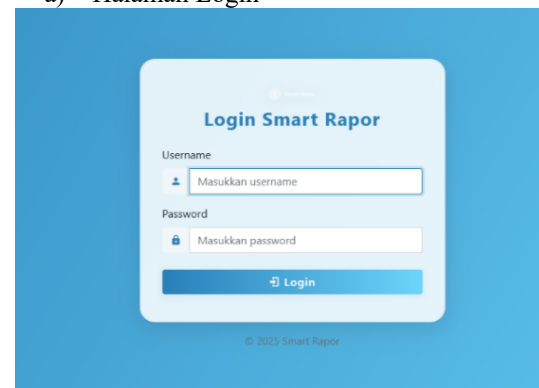
Gambar 6. Halaman Login
