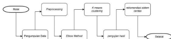
Gambar 1. Tahapan Penelitian
