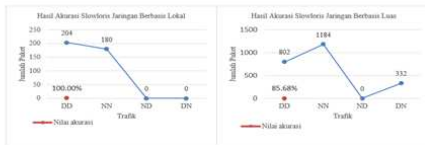
Gambar 12. Hasil Akurasi Serangan Slowloris di Jaringan Berbasis Lokal dan Luas
