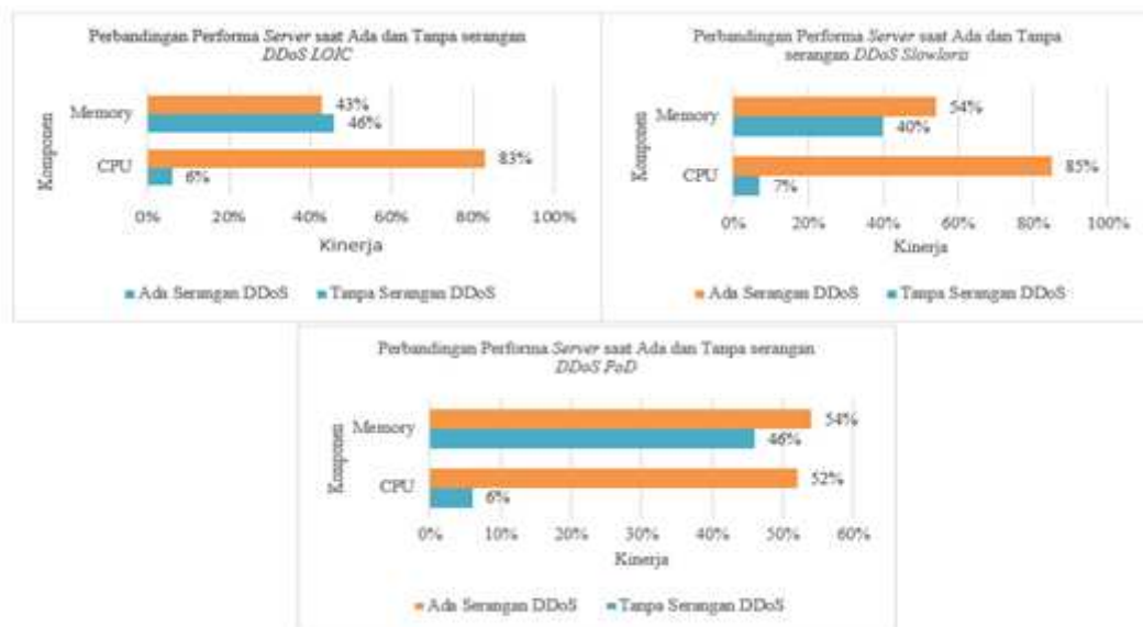
Gambar 14. Performa Web Server dengan Beberapa tool DDoS Saat Terjadi Serangan
