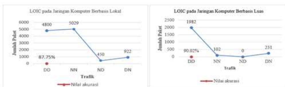
Gambar 11. Hasil Akurasi Serangan LOIC di Jaringan Komputer Berbasis Lokal dan Luas
