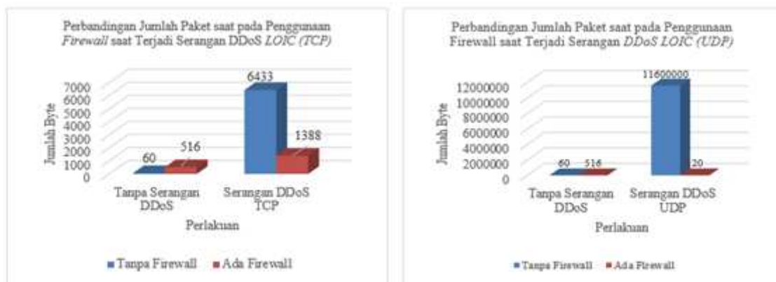
Gambar 23. Perbandingan Jumlah Byte sebelum dan setelah ada firewall pada DDoS LOIC pada TCP dan UDP
