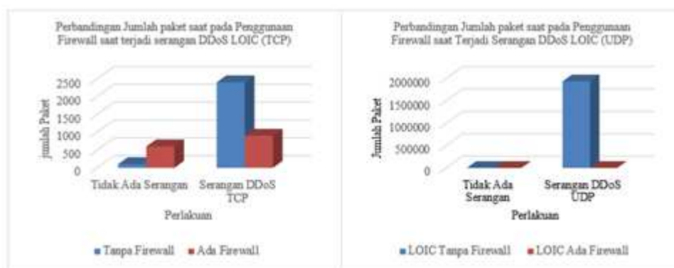
Gambar 21. Perbandingan sebelum dan setelah ada firewall pada DDoS LOIC pada TCP dan UDP
