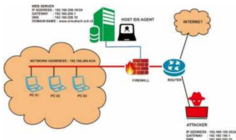
Gambar 4. Topologi Jaringan dan pengalamatan IP
