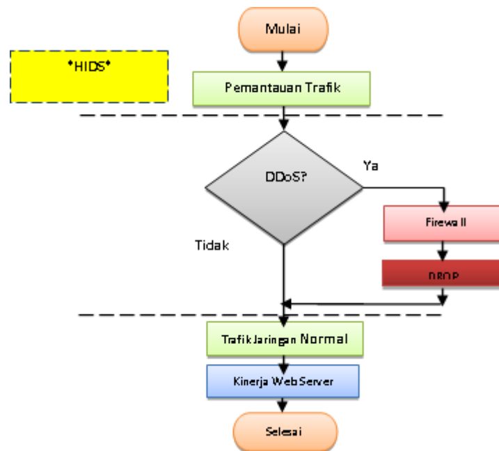
Gambar 3. Alur Metode HIDS pada DDoS
