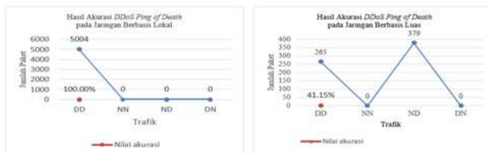
Gambar 13. Hasil Akurasi Serangan PoD di Jaringan Berbasis Lokal dan Luas
