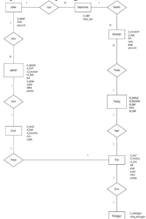
Gambar 2. ERD
