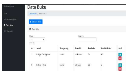
Gambar 4. Halaman Buku
