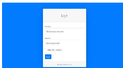
Gambar 1. Halaman Login
