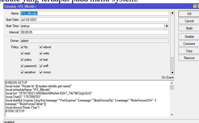
Gambar 2.5 Koneksi Mikrotik ke Telegram
