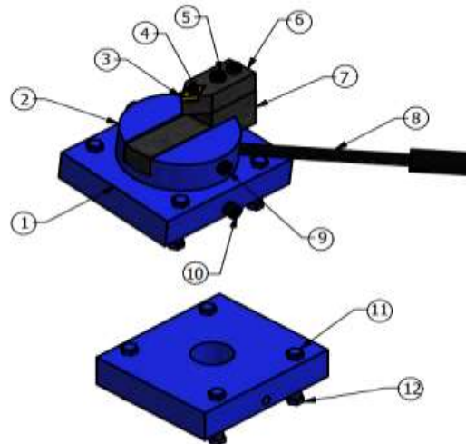
Gambar 1. Perencanaan Alat
