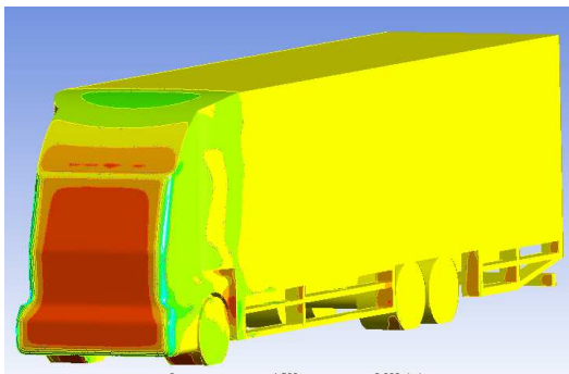
Gambar 7. Pressure countur truk full angin pada kecepatan 20 km/jam.
