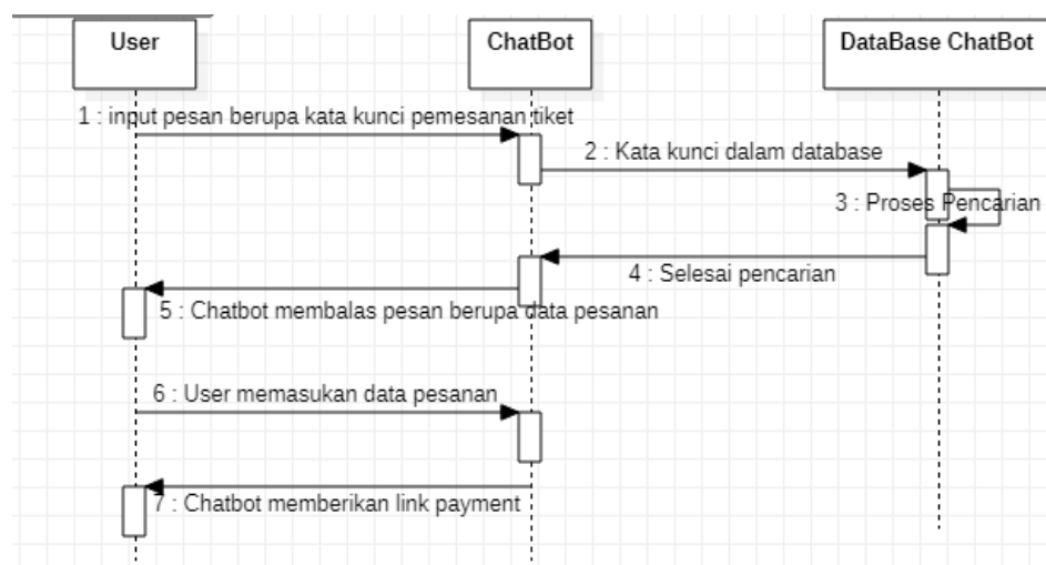
Gambar 6. Sequance Diagram Pemesanan Tiket
