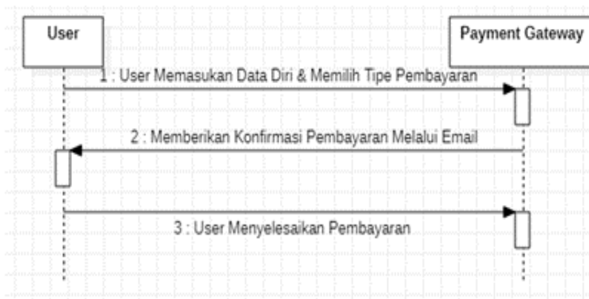
Gambar 7. Sequance Diagram Pembayaran Tiket
