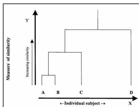
Gambar 1. Contoh Dendrogram
