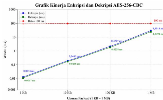
Gambar 3. Perbandingan waktu enkripsi dan dekripsi AES-256-CBC pada empat ukuran payload; seluruh nilai berada di bawah ambang persepsi 100 ms.
