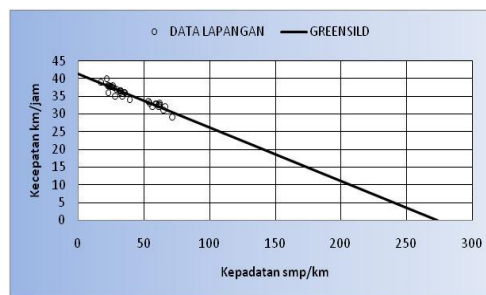
Gambar 2. Grafik Hubungan Kecepatan Dan Kepadatan Model Greenshield
