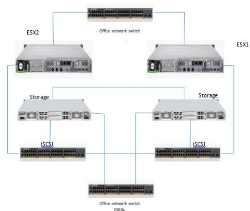
Gambar 1. Topologi VMware dan Storage
