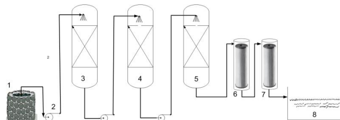
Gambar 1. Rangkaian peralatan pengolahan air payau
