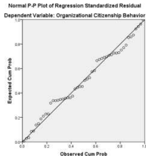
Gambar 4.1. P-plot
