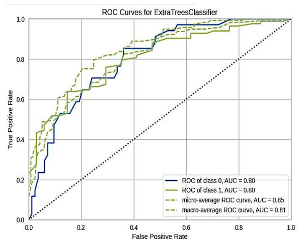
Gambar 5. Kurva AUC/ROC
