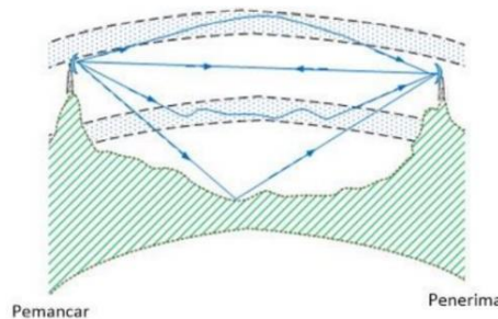
Gambar 7. Refraksi
