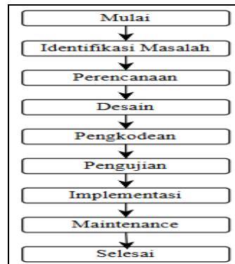
Gambar 1. Desain Penelitian
