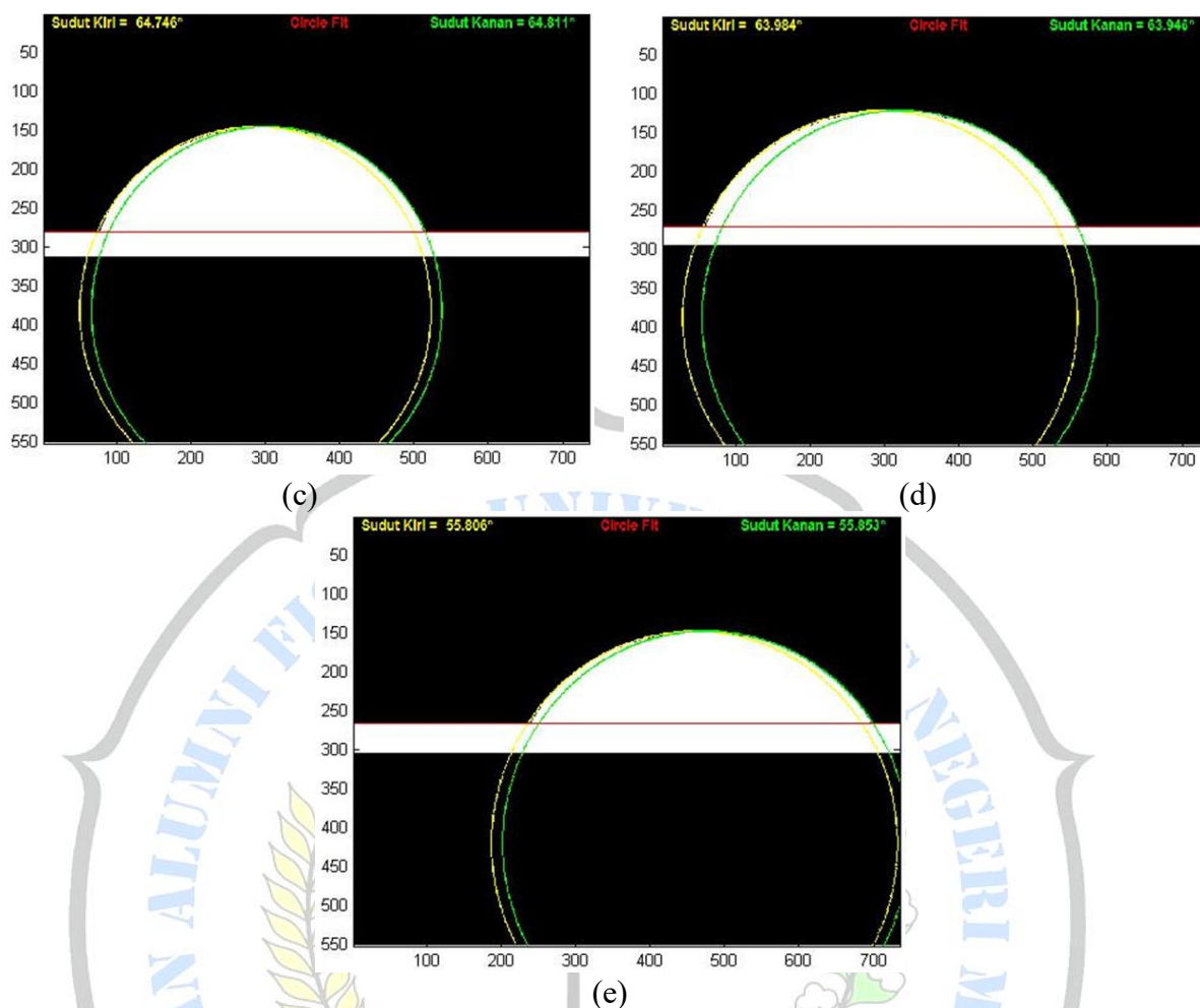
Gambar 1. Hasil pengukuran nilai sudut kontak lapisan Ps: (a) 0 menit, (b) 30 menit, (c) 60 menit, (d) 90 menit, (e) 120 menit
