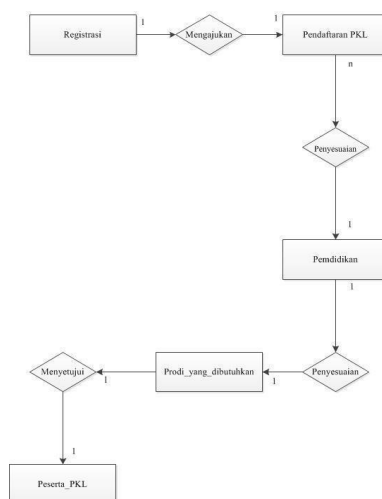
Gambar 3.7 ERD
