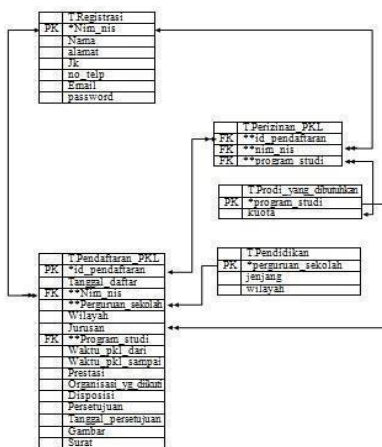
Gambar 3.6 Relasi Tabel
