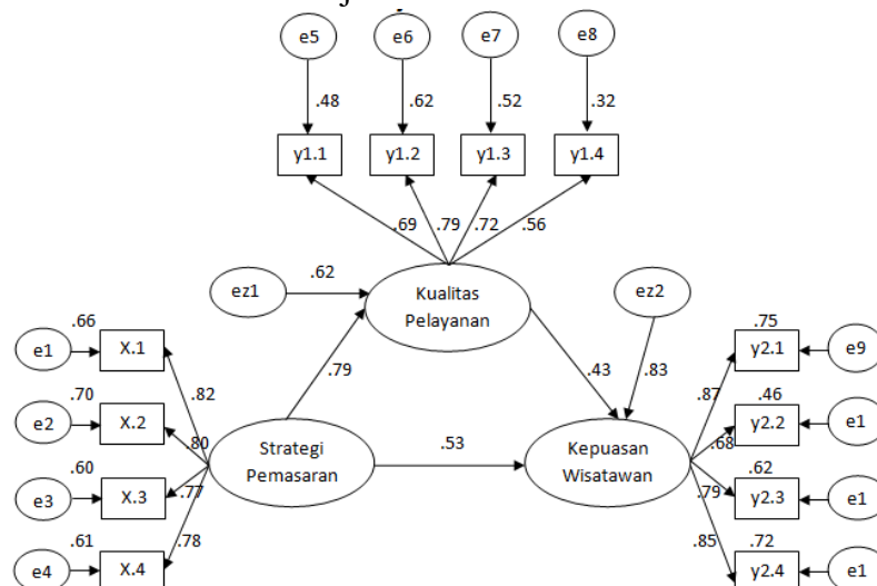
Gambar 2. Hasil Uji Model Persamaan Struktural
