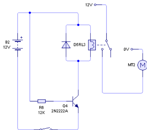
Gambar 9. Pompa DC
