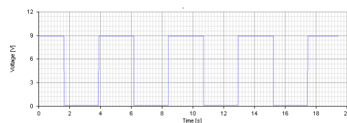
Gambar 3. Bentuk Gelombang Kotak
