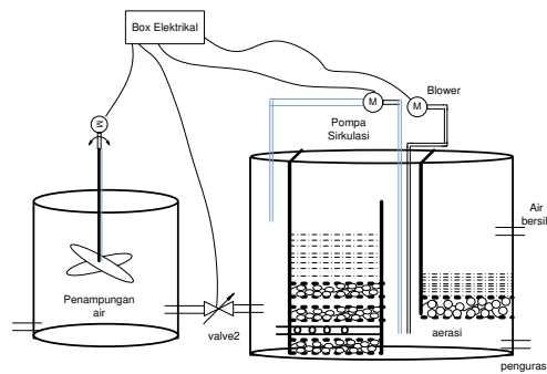
Gambar 7. Model Perancangan Alat
