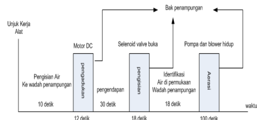
Gambar 11. Unjuk Kerja Peralatan
