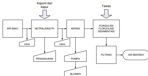
Gambar 1. Proses Pengolahan Air Sederhana
