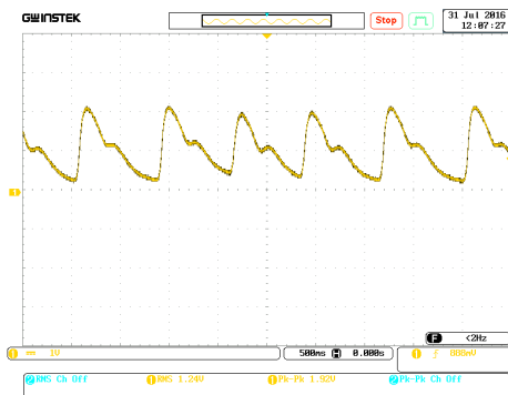
Gambar 4. Sinyal PPG dari pengukuran sensor
