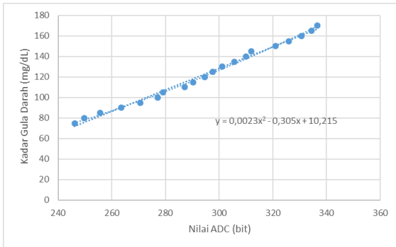
Gambar 5. Hubungan antara nilai ADC dengan Kadar gula darah
