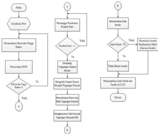
Gambar 3. Flowchart Pengolahan Sinyal pada Mikrokontroler
