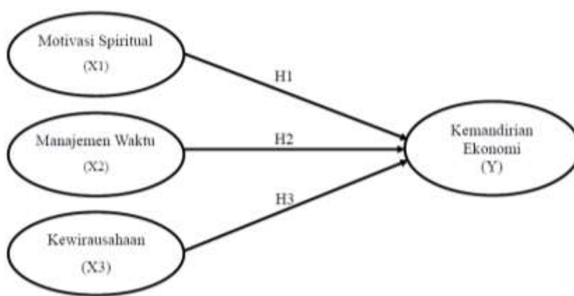
Gambar 1. Kerangka Penelitian
