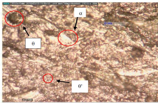
Gambar 12 Spesimen di heat treatment dengan suhu 150 °C waktu tahan 60 Menit
