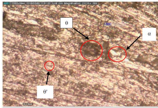
Gambar 11 Spesimen di heat treatment dengan suhu 100 °C waktu tahan 120 Menit
