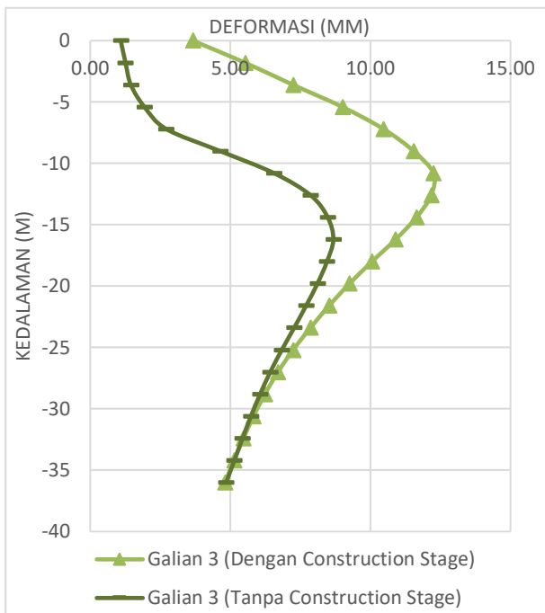
Gambar 17. Perbandingan hasil deformasi dinding antara analisis construction stage dan analisis konvensional pada galian tahap 3
