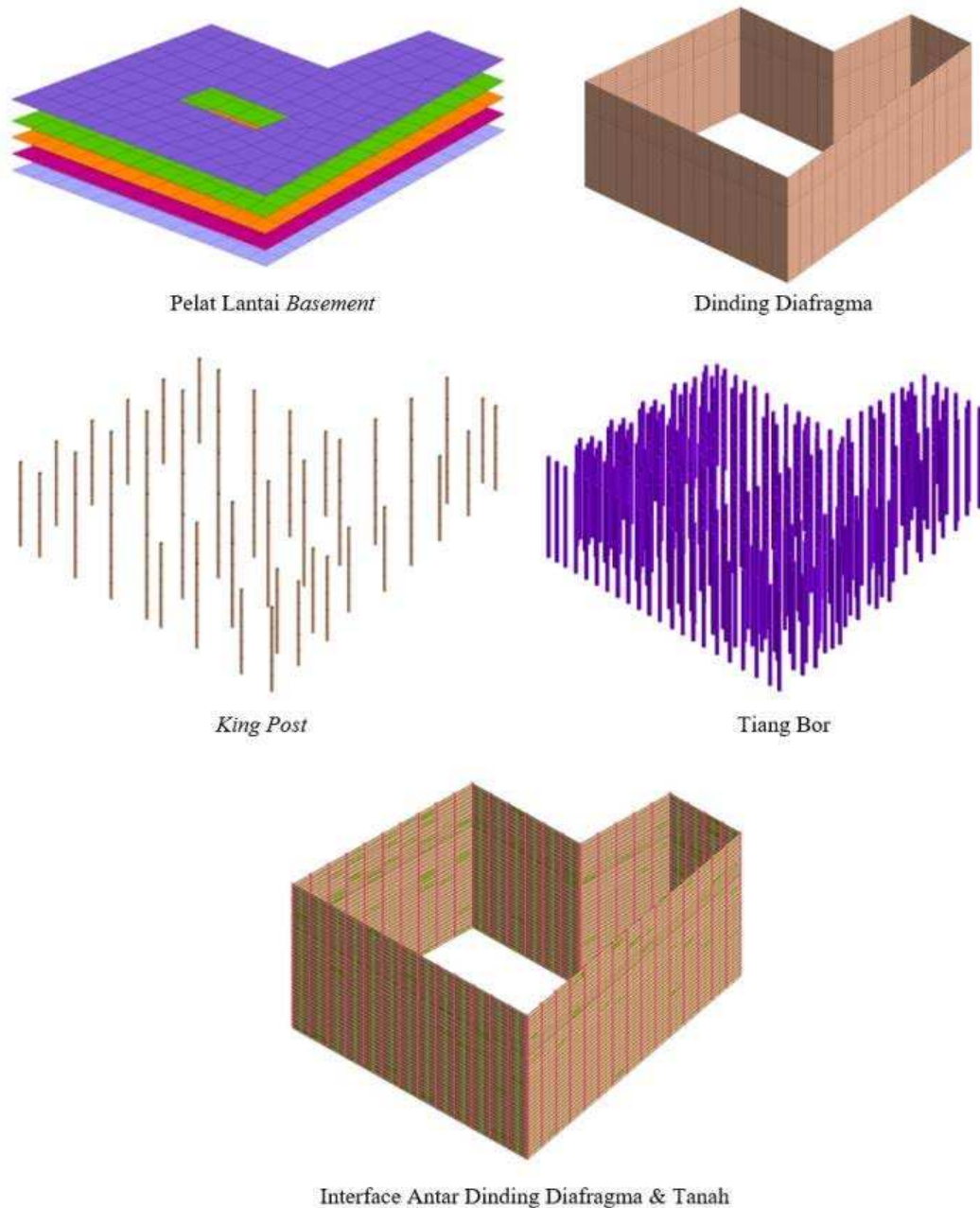
Gambar 7. Hasil meshing untuk dinding diafragma dan struktur basement
