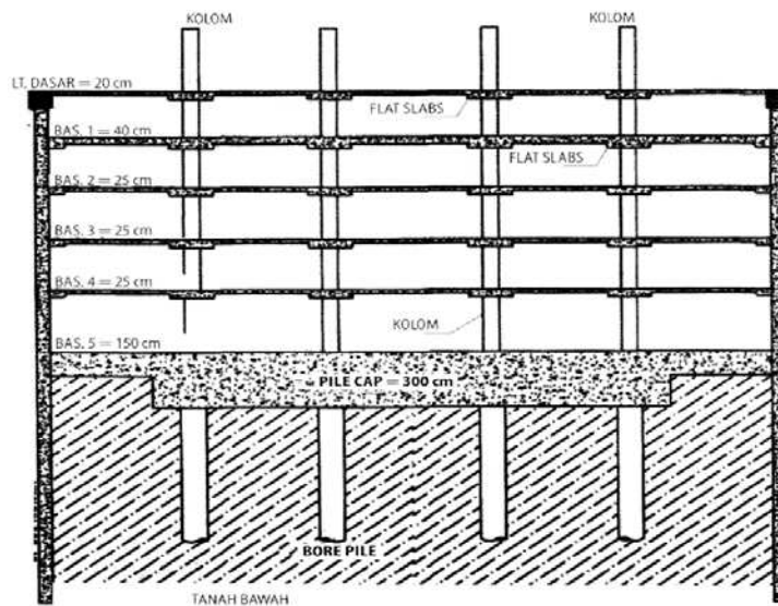
Gambar 3. Potongan basement dengan metode top-down (Sumber: Mistra, 2012)
