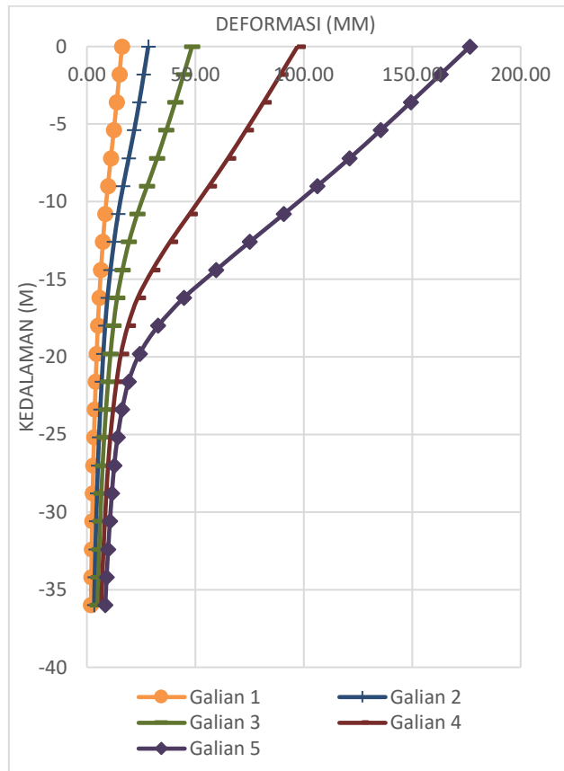
Gambar 12. Grafik deformasi dinding (tanpa pelat) pada tiap tahap galian
