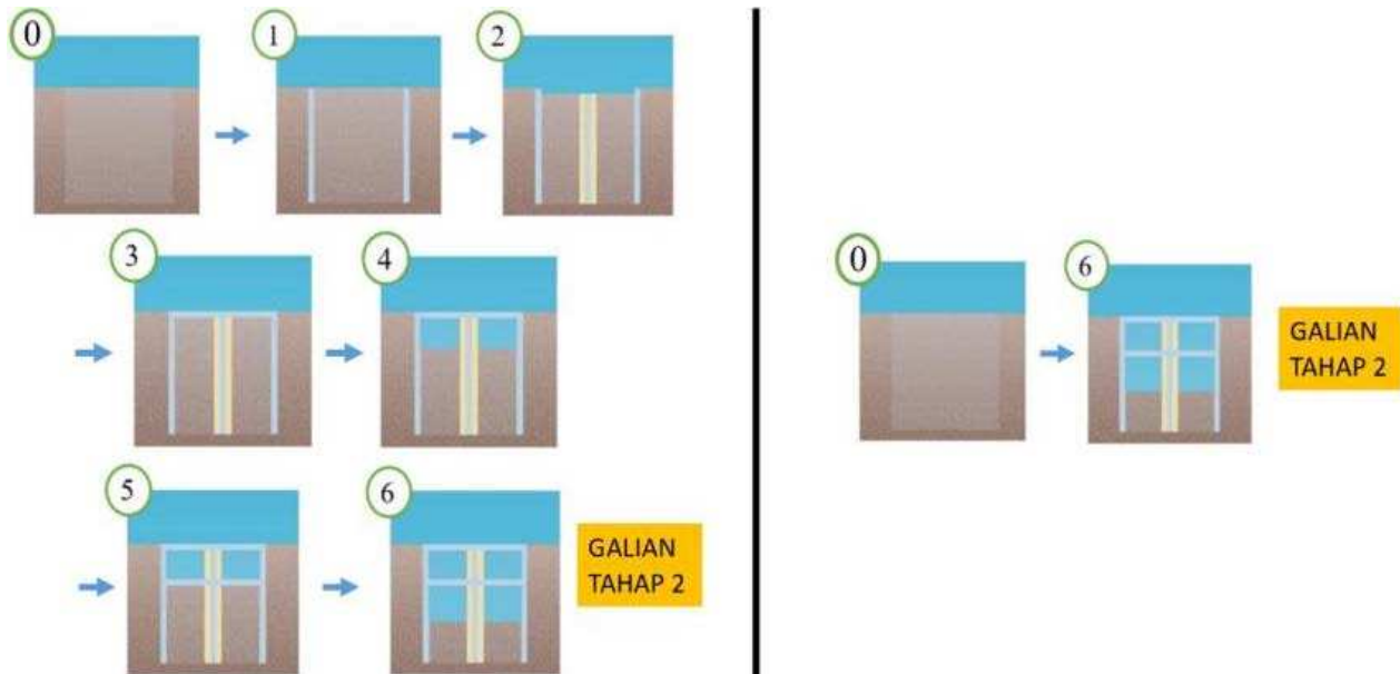
Gambar 1. Ilustrasi analisis construction stage (kiri) dan analisis konvensional (kanan)
