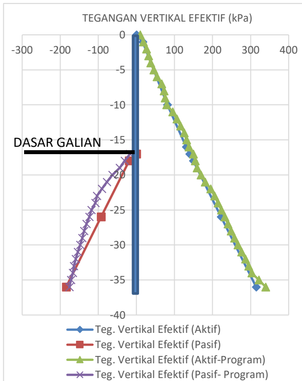
Gambar 8. Tegangan Vertikal Efektif (Program Vs Hitungan Manual)
