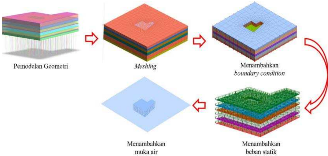
Gambar 5. Tahapan pemodelan 3D pada MIDAS GTS NX
