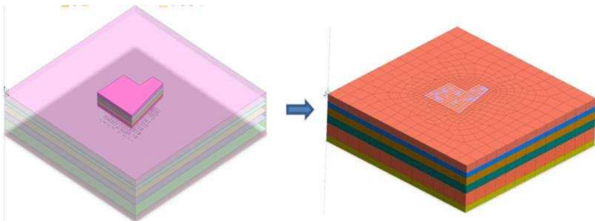
Gambar 6. Pemodelan geometri dan meshing tanah
