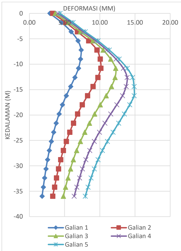
Gambar 11. Grafik deformasi dinding (dengan pelat) pada tiap tahap galian
