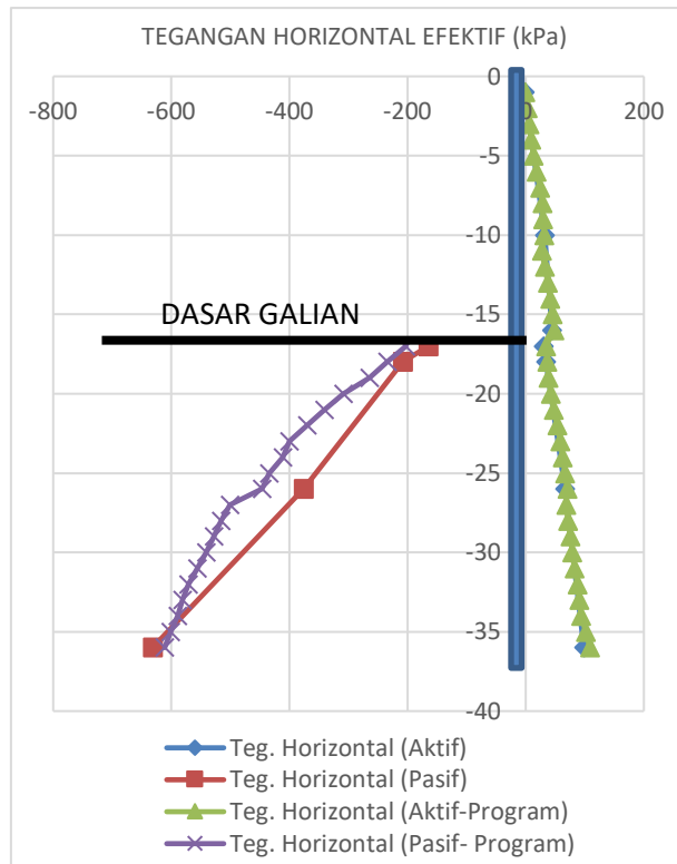
Gambar 9 Tegangan Horizontal Efektif (Program Vs Hitungan Manual)
