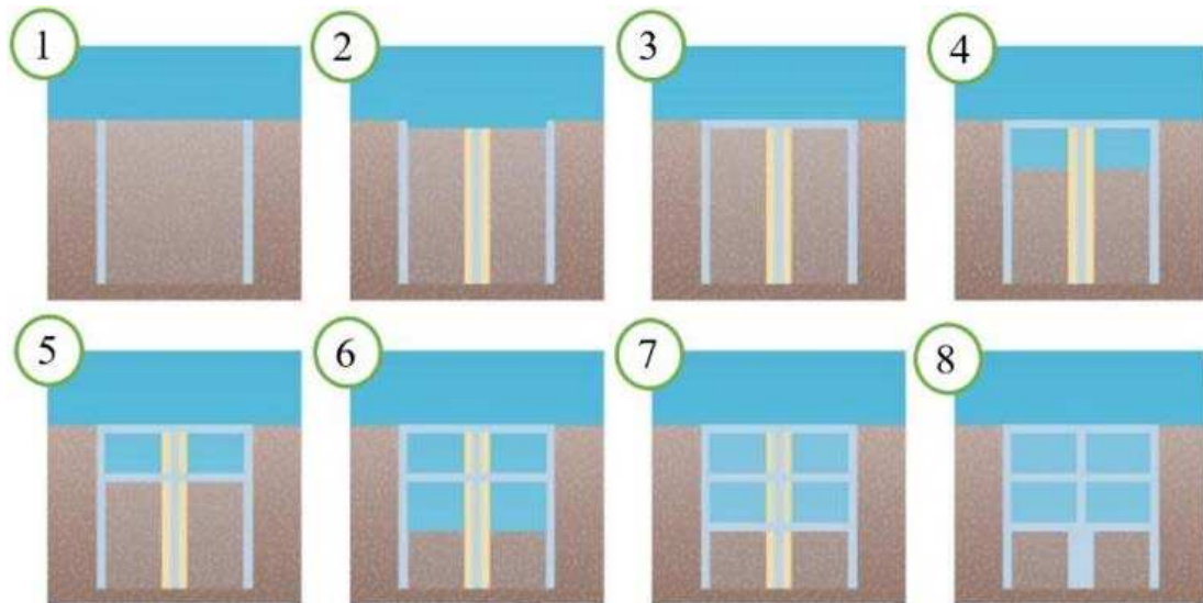
Gambar 2. Pekerjaan basement dengan sistem top-down
