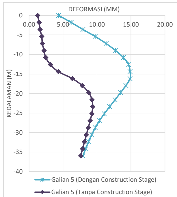
Gambar 18. Perbandingan hasil deformasi dinding antara analisis construction stage dan analisis konvensional pada galian tahap 5
