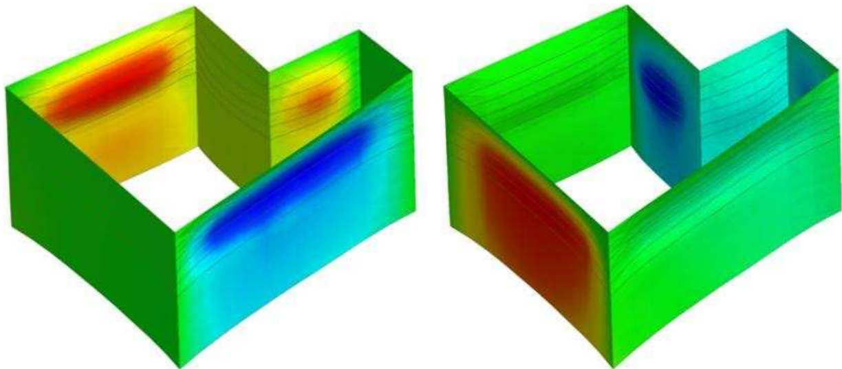
Gambar 10. Deformasi dinding arah x (kiri) dan arah y (kanan)
