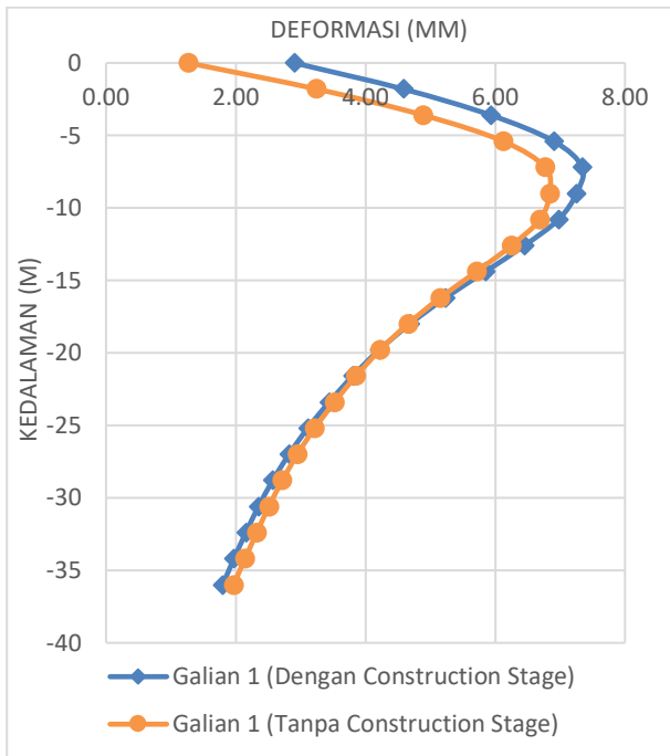
Gambar 15. Perbandingan hasil deformasi dinding antara analisis construction stage dan analisis konvensional pada galian tahap 1
