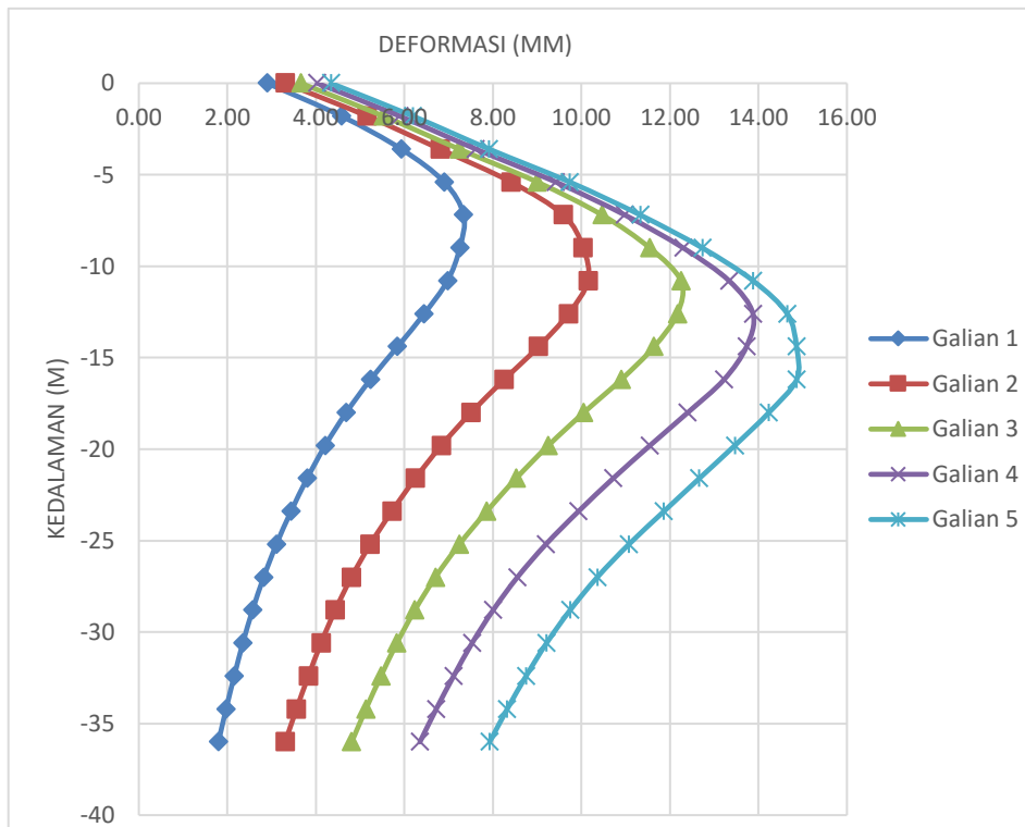
Gambar 13. Hasil deformasi dinding dengan analisis construction stage
