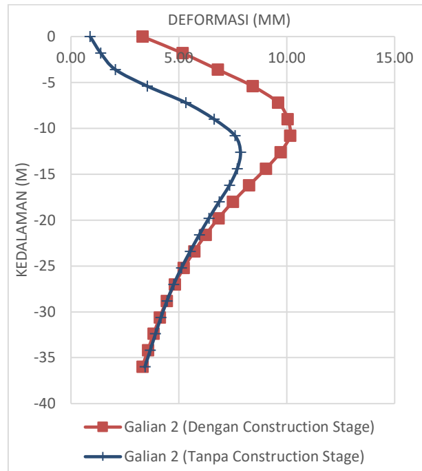
Gambar 16. Perbandingan hasil deformasi dinding antara analisis construction stage dan analisis konvensional pada galian tahap 2
