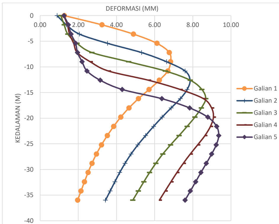
Gambar 14. Hasil deformasi dinding dengan analisis konvensional
