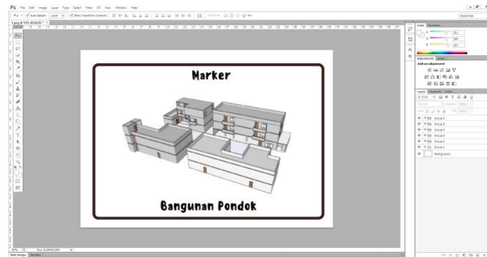
Gambar 8. Pembuatan Marker
