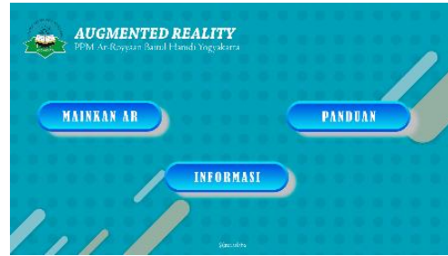
Gambar 13. Halaman Menu
