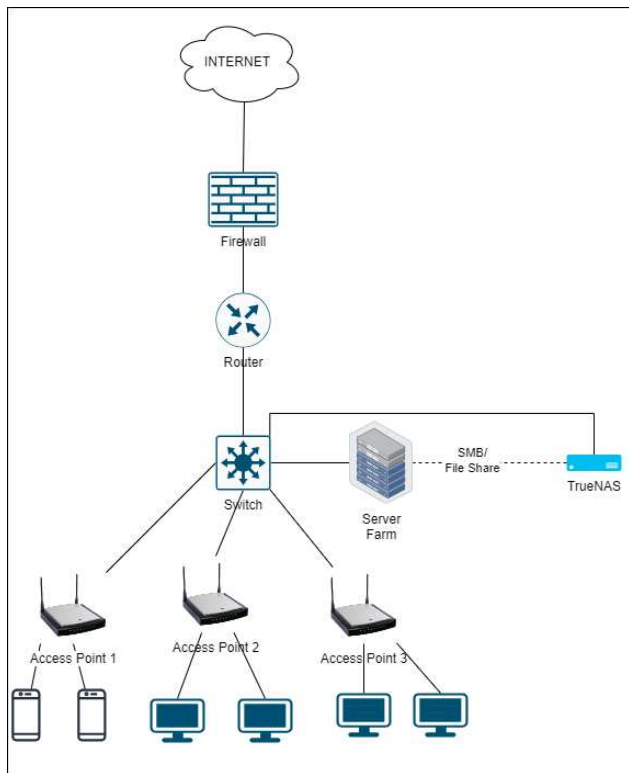
Gambar 4. Topologi saat ini
