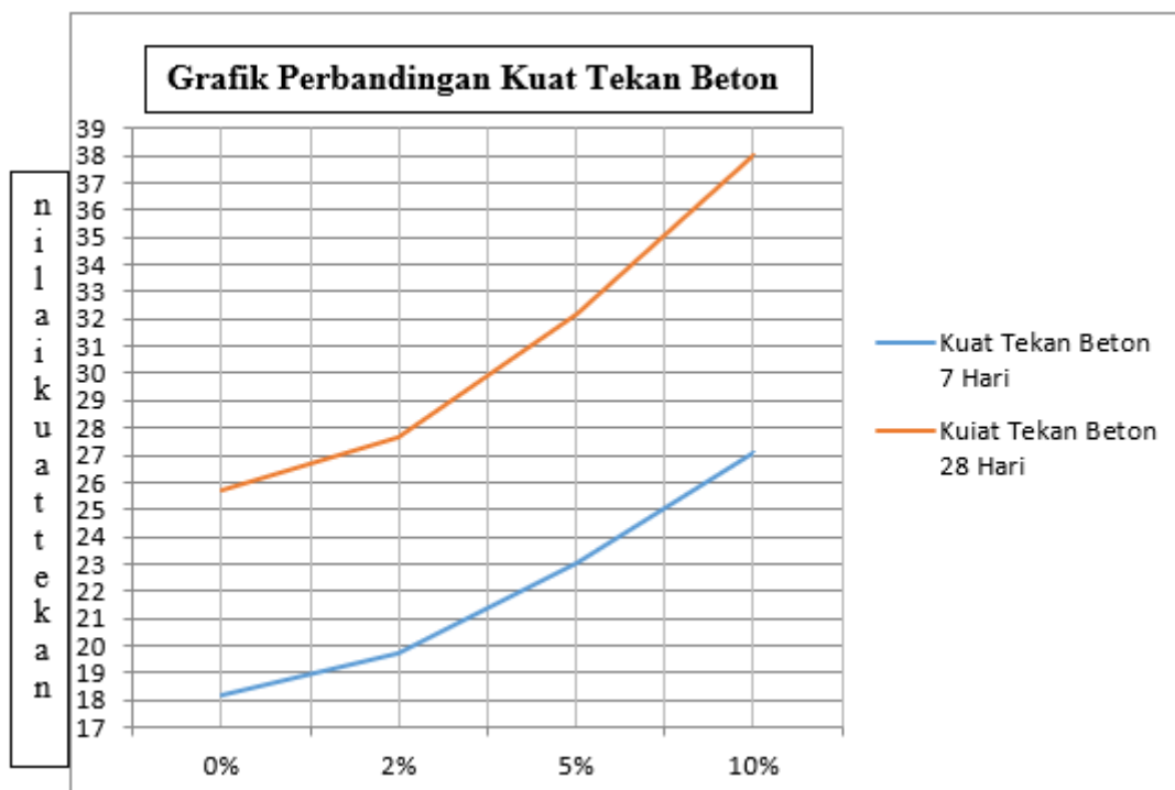
Gambar 5. Nilai kuat tekan beton normal dan beton menggunakan bahan tambah ADDITON H.E. umur 28 hari
