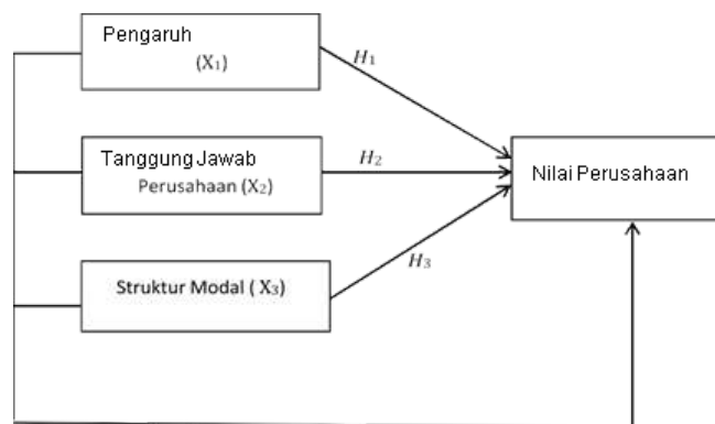
Gambar 1. Kerangka Berpikir
