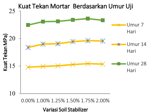
Gambar 3. Grafik Kuat Tekan Mortar Pasir Sungai Gebang umur 7, 14, dan 28 hari.
