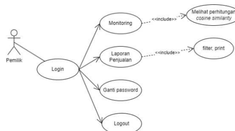
Gambar 4. 2 Use Case Diagram Pemilik Toko
