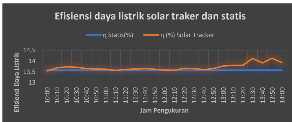
Gambar 8. Efisiensi daya listrik pada posisi solar traker dan posisi statis
