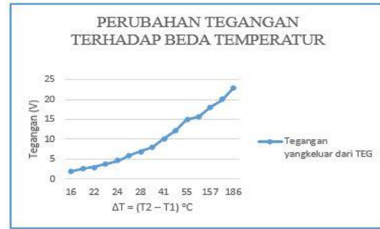
Gambar 6. Grafik Pengujian Perubahan Tegangan Terhadap Beda Temperatur
