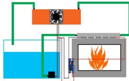
Gambar 4. Skema termoelektrik
