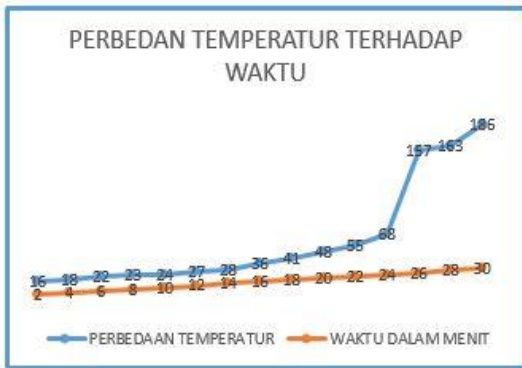
Gambar 4.16. Grafik hasil pengujian perbedaan temperatur terhadap waktu
