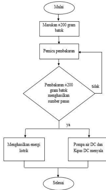
Gambar 3. Diagram alir cara kerja alat
