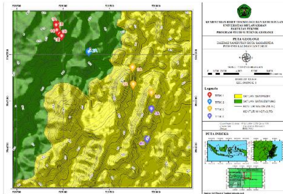
Gambar 4.7 Peta Geologi
