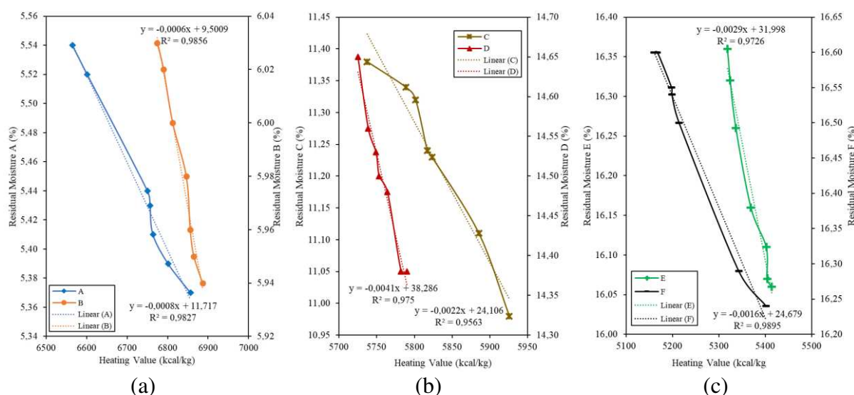
Gambar 1. Korelasi nilai Heating Value (HV) dengan Residual Moisture (RM) batubara HCV(a), MCV(b), dan LCV(c)
