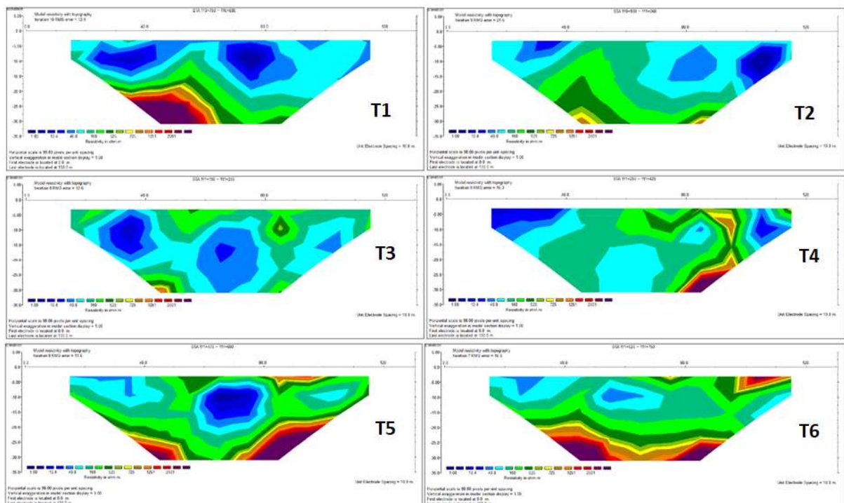
Gambar 5. Hasil interpretasi geolistrik tiap lintasan
