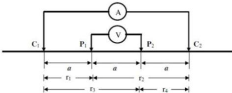
Gambar 1. Konfigurasi Wenner-Alpha
