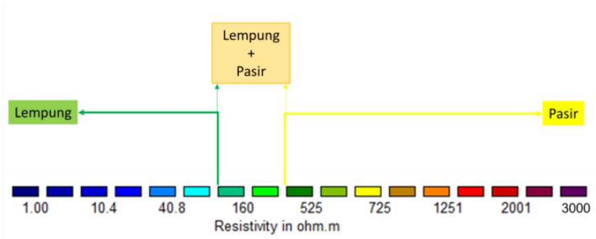
Gambar 4. Interpretasi nilai resistivitas lapisan tanah
