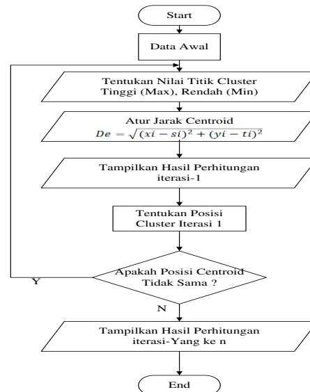
Gambar 3.1. Algoritma Sistem
