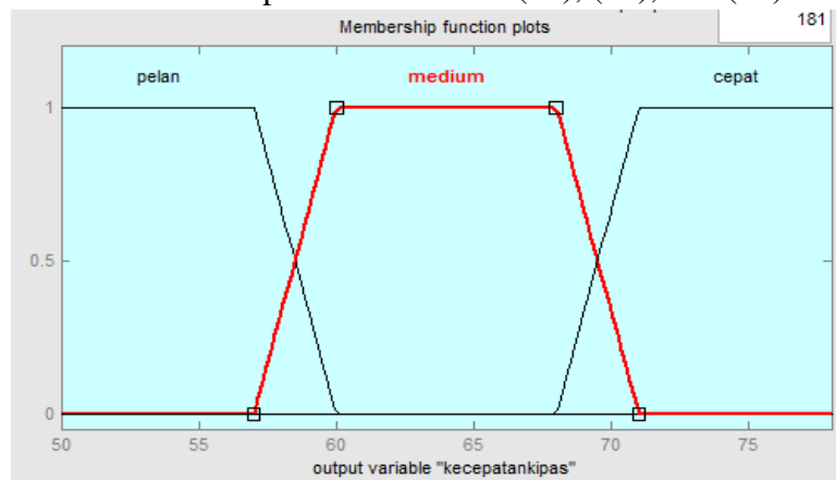
Gambar 5. Himpunan Fuzzy Variabel Kipas
