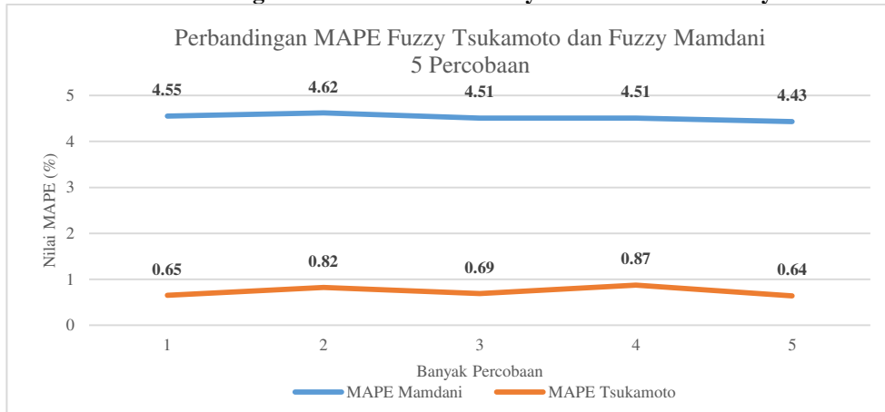
Gambar 9. Perbandingan MAPE Fuzzy Tsukamoto dan Fuzzy Mamdani
