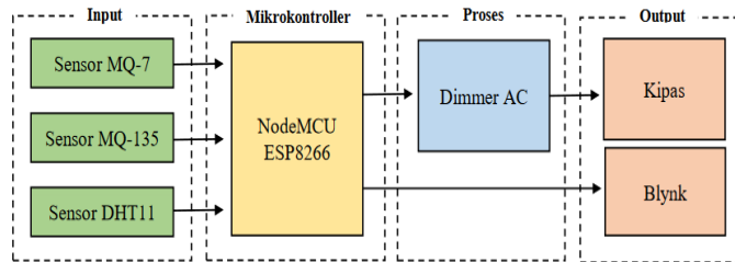
Gambar 2. Diagram Perangkat Keras Sistem Kendali Exhaust Fan
