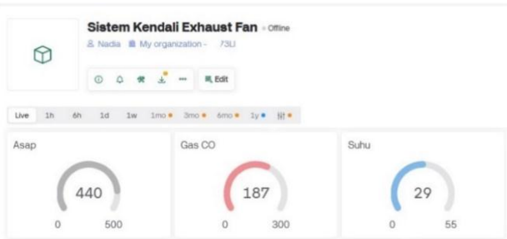
Gambar 7. Pembacaan Sensor dan Data Kecepatan Kipas Hasil dari Metode Fuzzy
