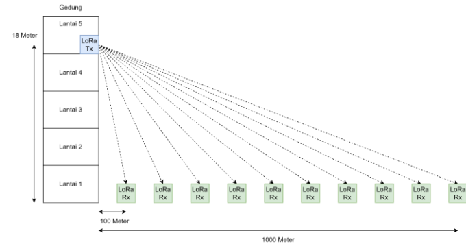
Gambar 14 Ilustrasi pengukuran nilai RSSI antara perangkat LoRa Tx dengan Rx
